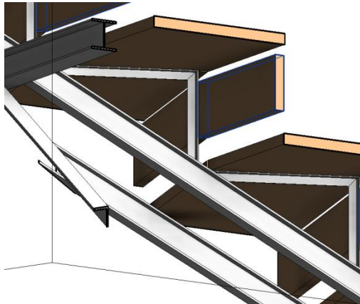
Figure9: Τρισδιάσταση απεικόνιση έδρασης καθισμάτων.
