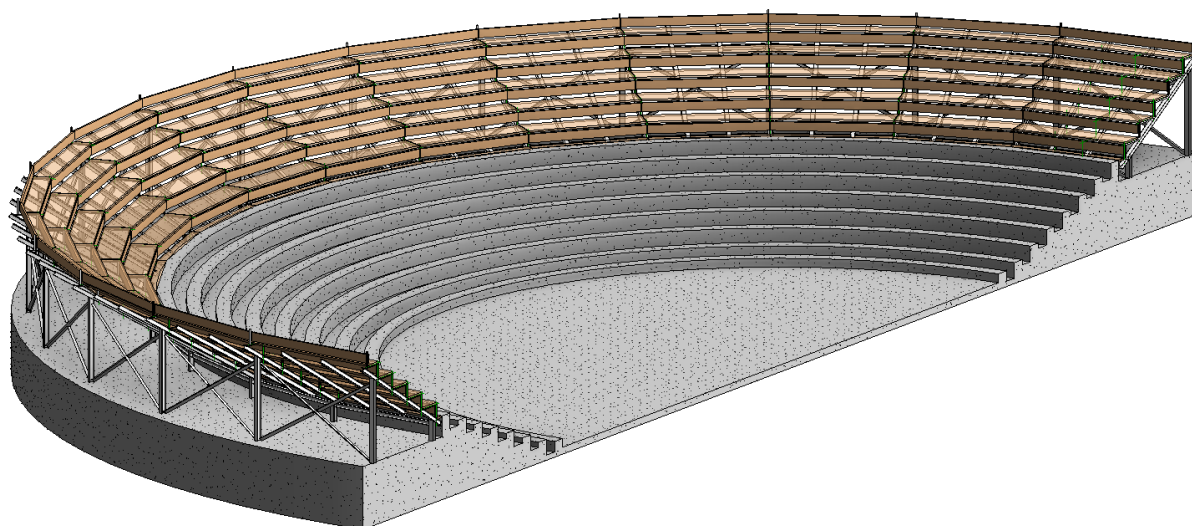
Εικόνα3: Τρισδιάστατη απεικόνιση των προστιθέμενων κερκίδων.
