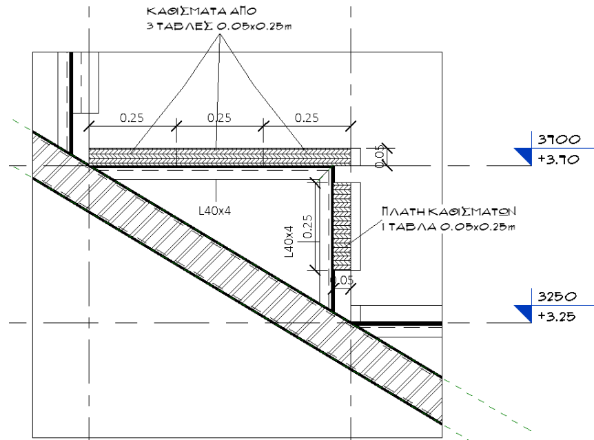
Figure 1: Λεπτομέρεια καθισμάτων.
