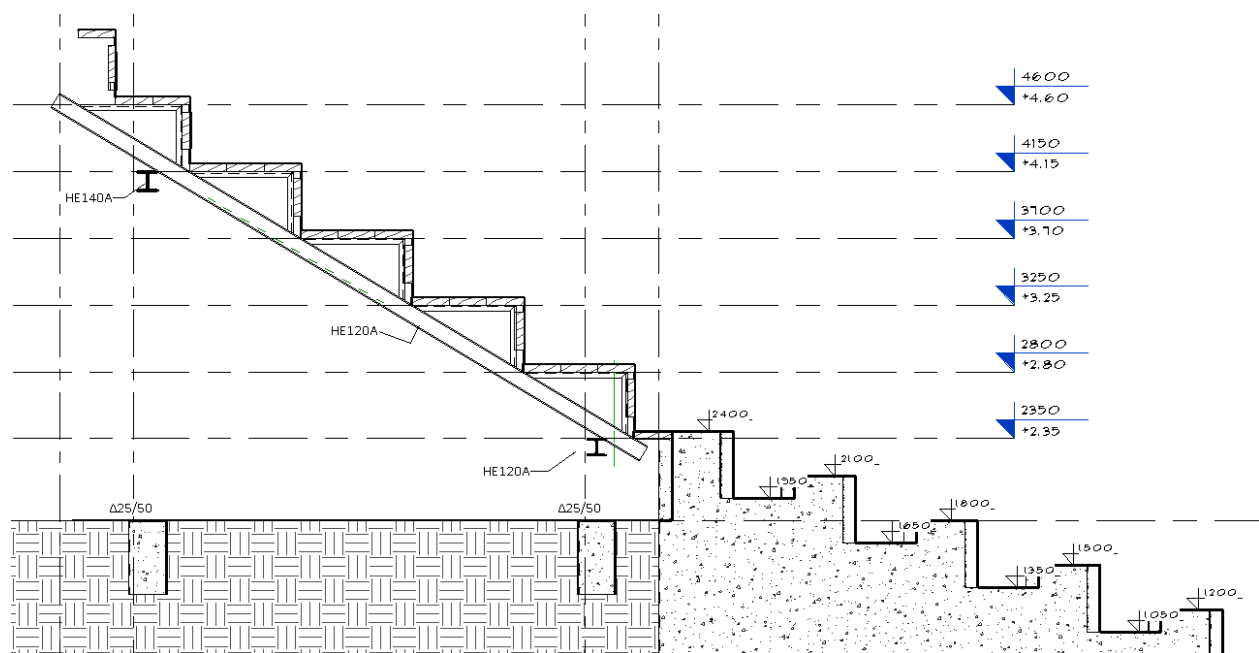
Εικόνα6: Οψη τυπικών πλαισίων χωρίς υποστρώματα.
