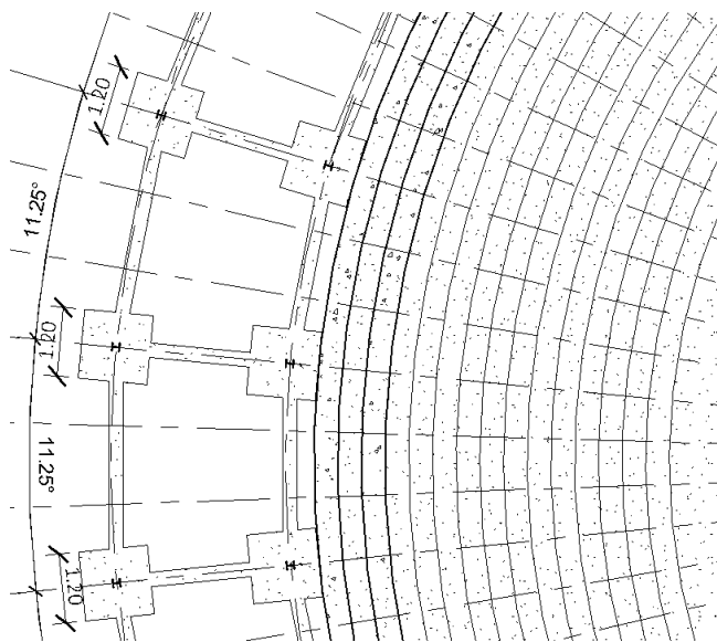
Εικόνα 4: Τμήμα κάτοψης του ξυλοτύπου θεμελίωσης.
