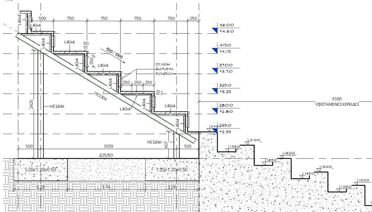
Εικόνα5: Οψη τυπικών πλαισίων με υποστρώματα.
